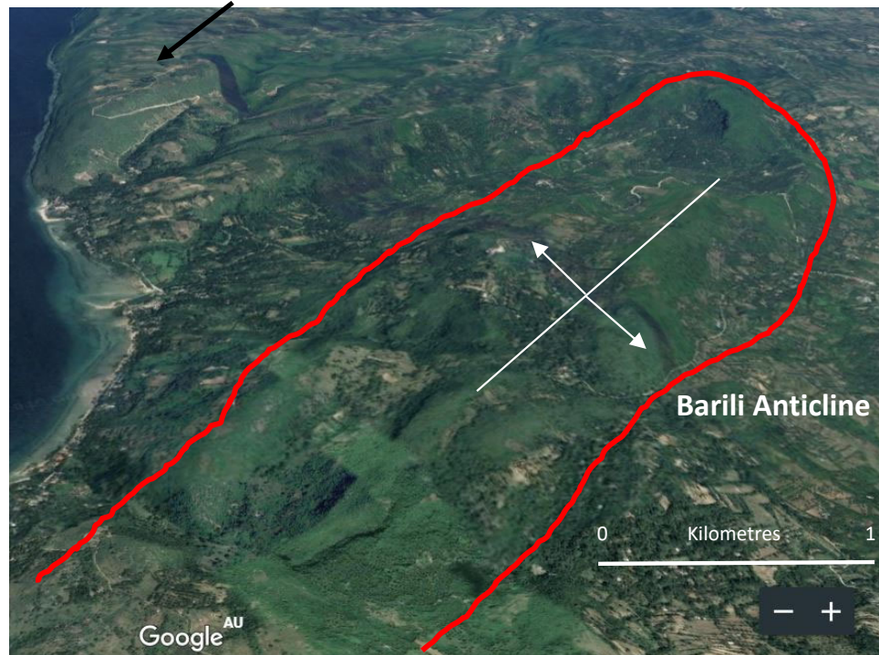
Pinamungahan Anticline
