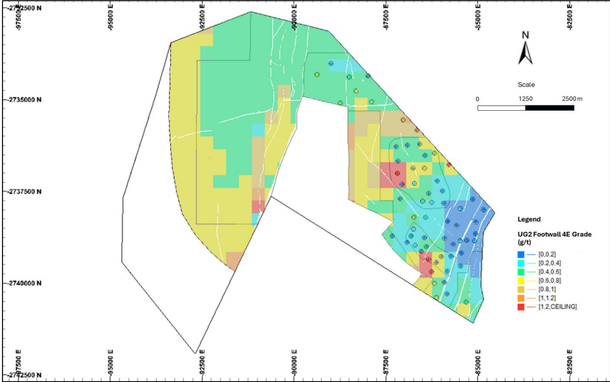
Figure 2: UG2 Footwall 4E Mineralisation Model (g/t)
