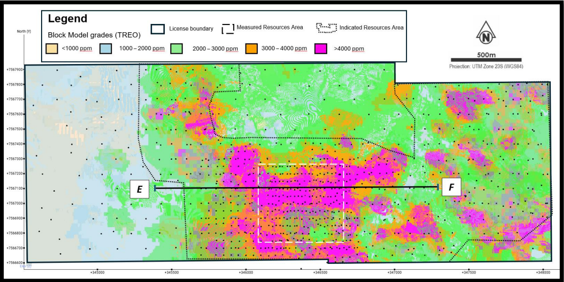
Capão do Mel - Plan view
